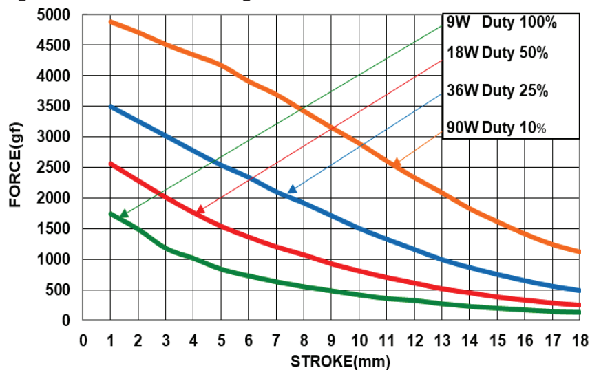
Kraft-Wege-Diagramm / Stroke-Force-Diagram
